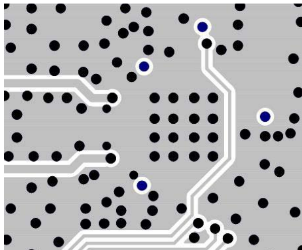
Inner Layer 4
